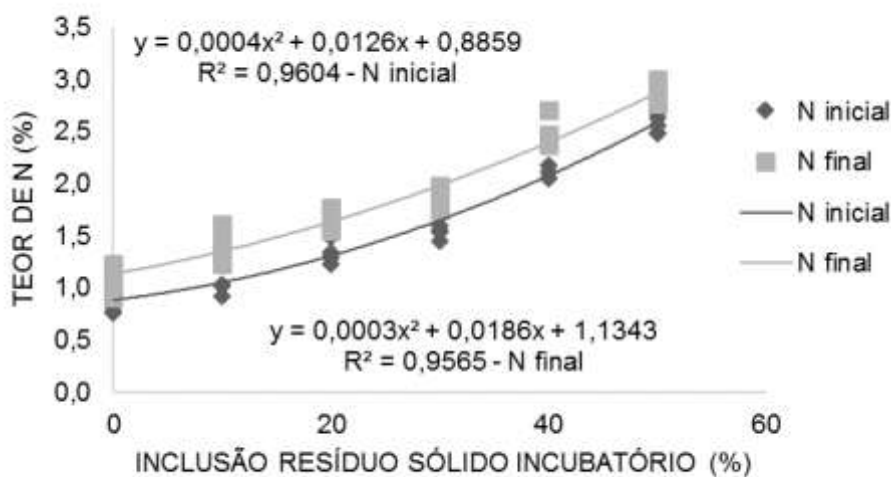
Figura 5- Teores de N (%) no material inicial e final da compostagem dos dejetos de ovinos e níveis crescentes de inclusão de resíduo sólido de incubatório.
