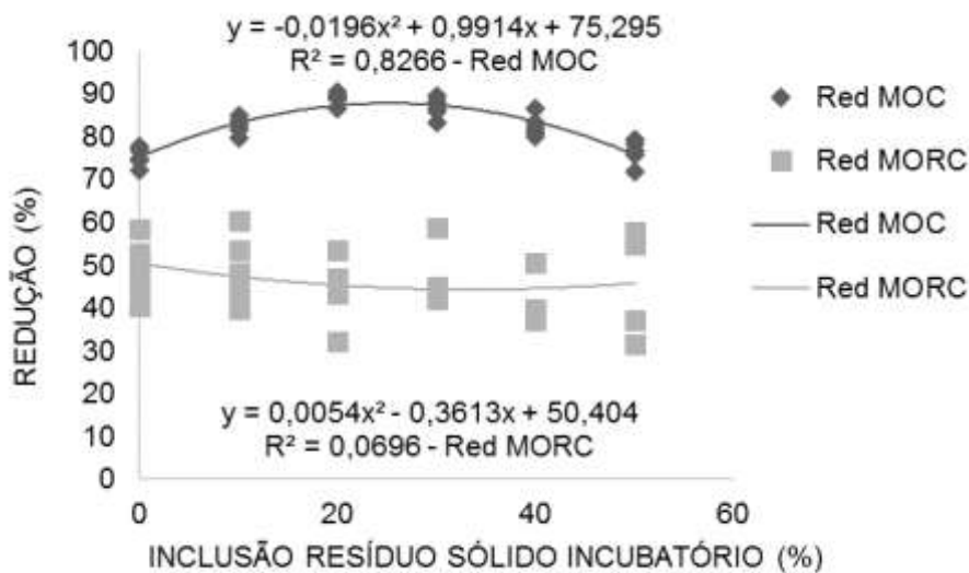
Figura 6- Reduções da matéria orgânica compostável (MOC) e matéria orgânica resistente à compostagem (MORC) a compostagem dos dejetos de ovinos e níveis crescentes de inclusão de resíduo sólido de incubatório.
